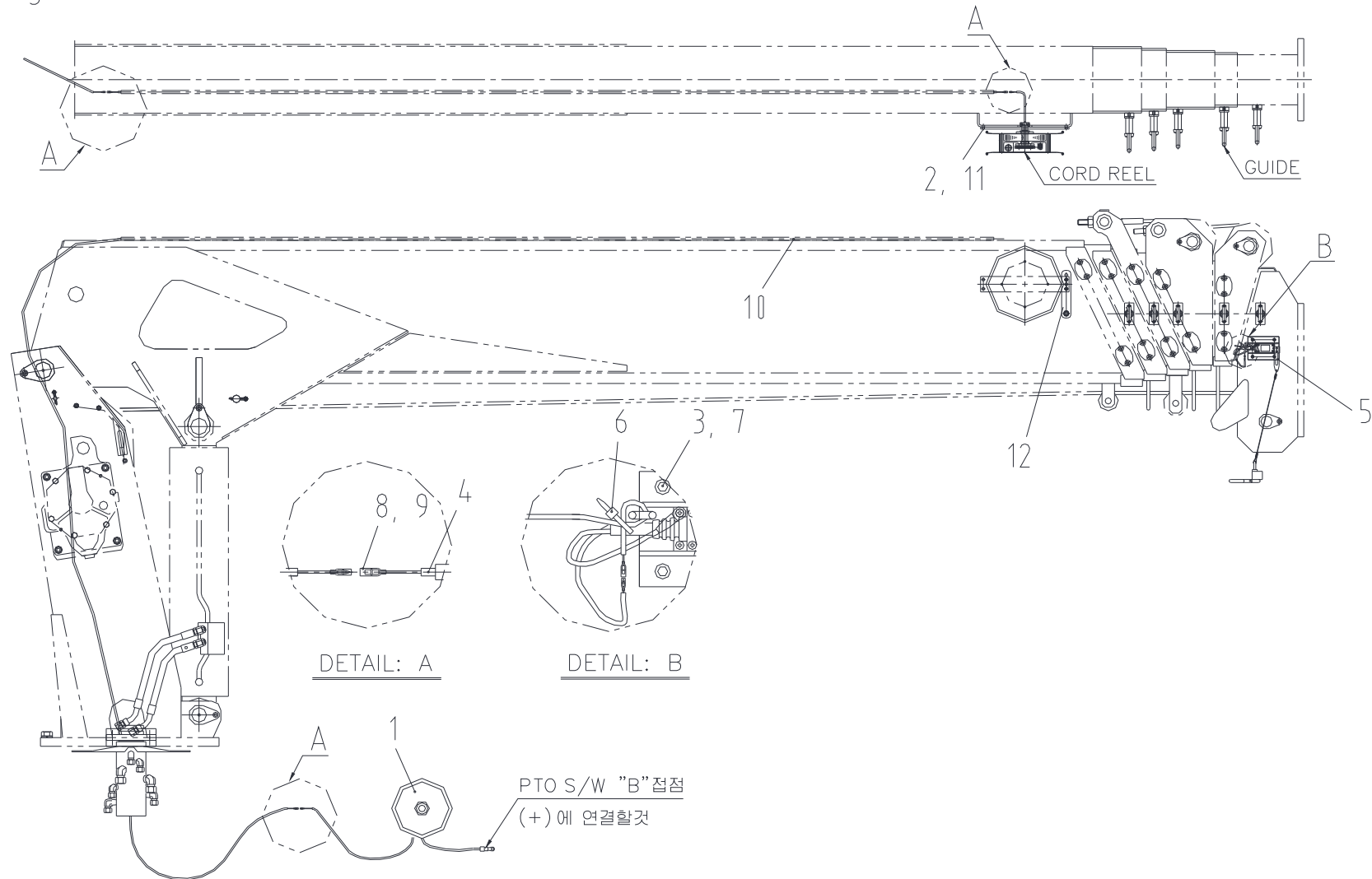
Fig. 13 과권방지장치 조립체
