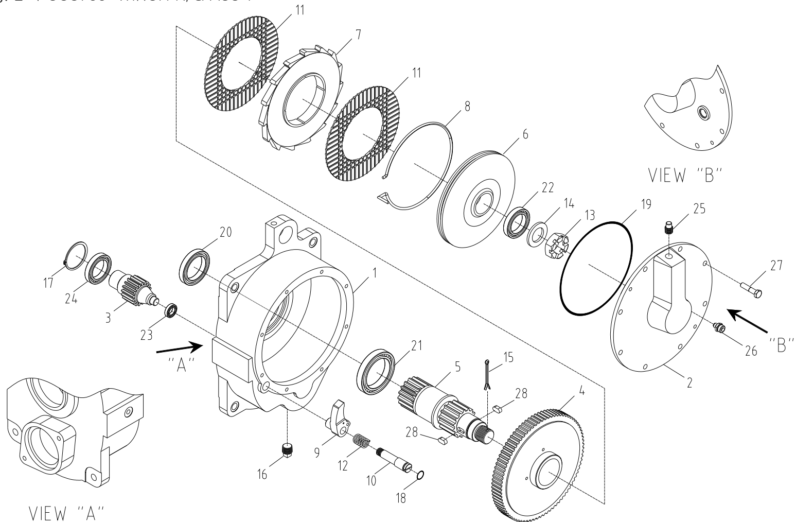
원치 감속기 조립체 Fig. 2-1 SCS736 WINCH R/G ASS'Y
