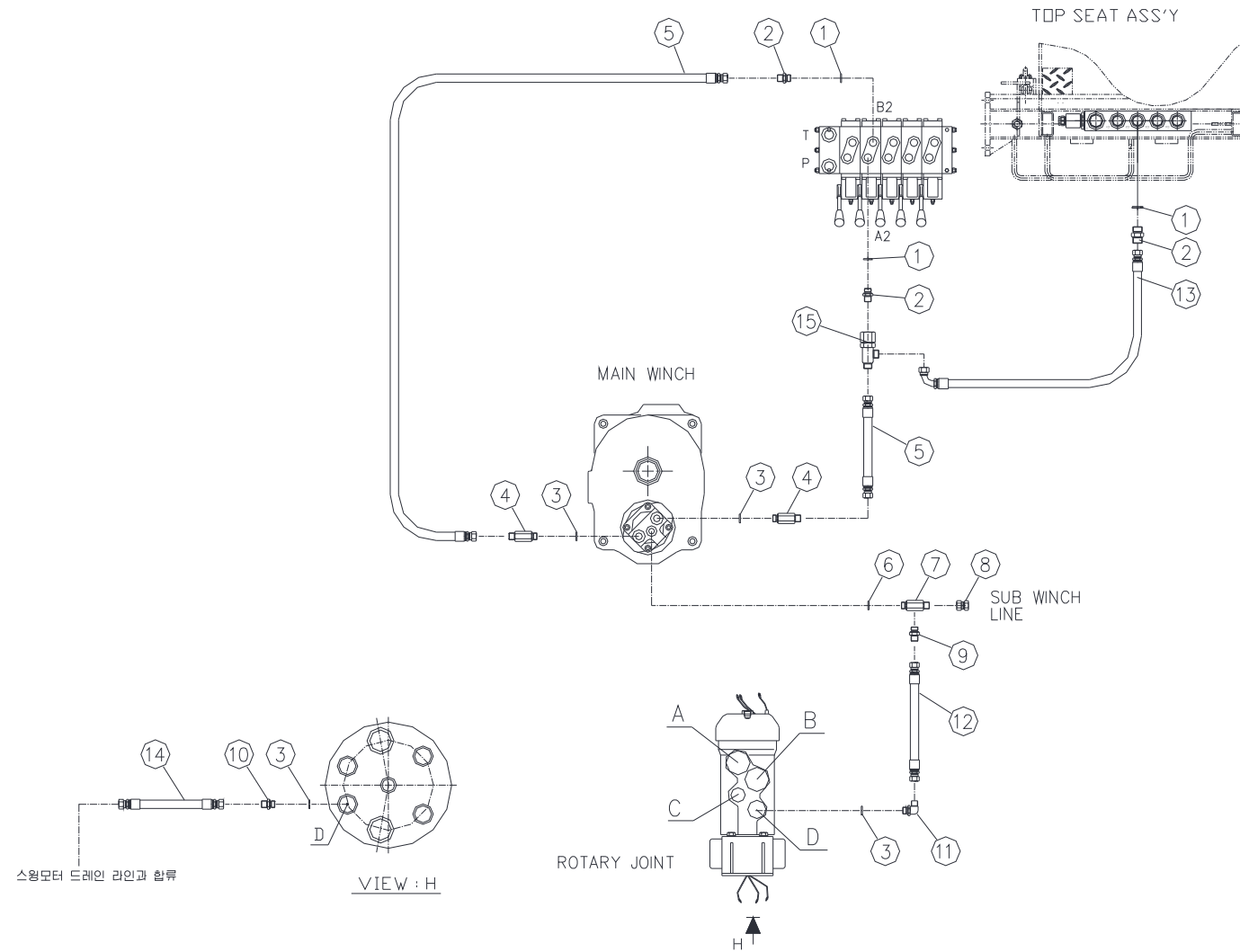
주 윈치 배관|탑형| Fig. 5-3 SCS736 MAIN WINCH PIPING(TOP)
