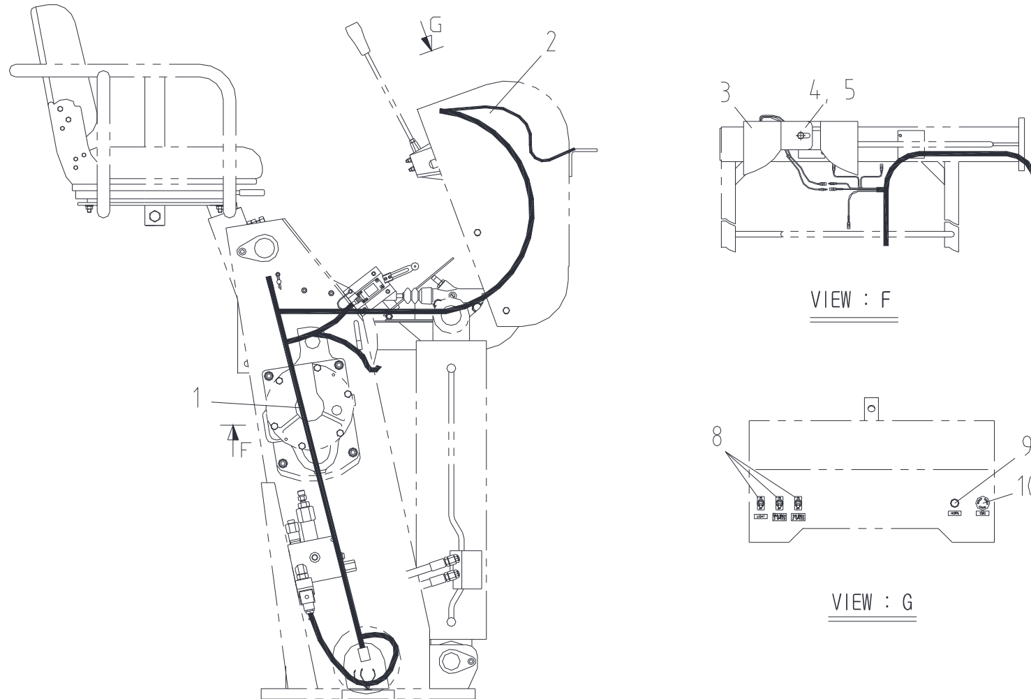
포스트 전선 Fig. 10-2 SCS736, SCS736L2 POST WIRING (TOP)
