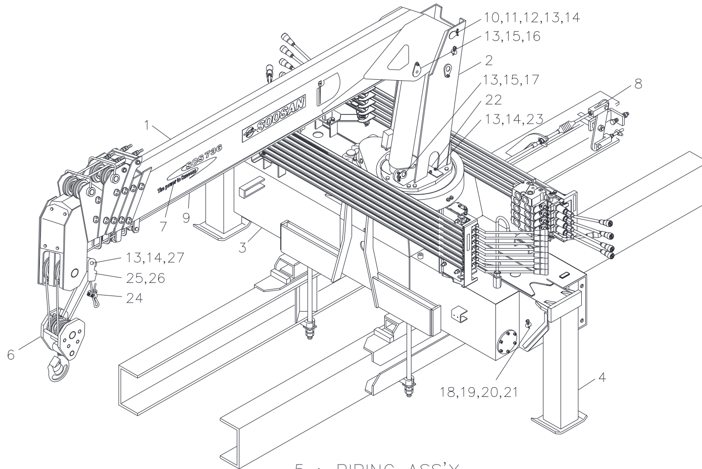
크레인 조립체 (표준형) Fig. 0 SCS736 CRANE ASS'Y (STD)
