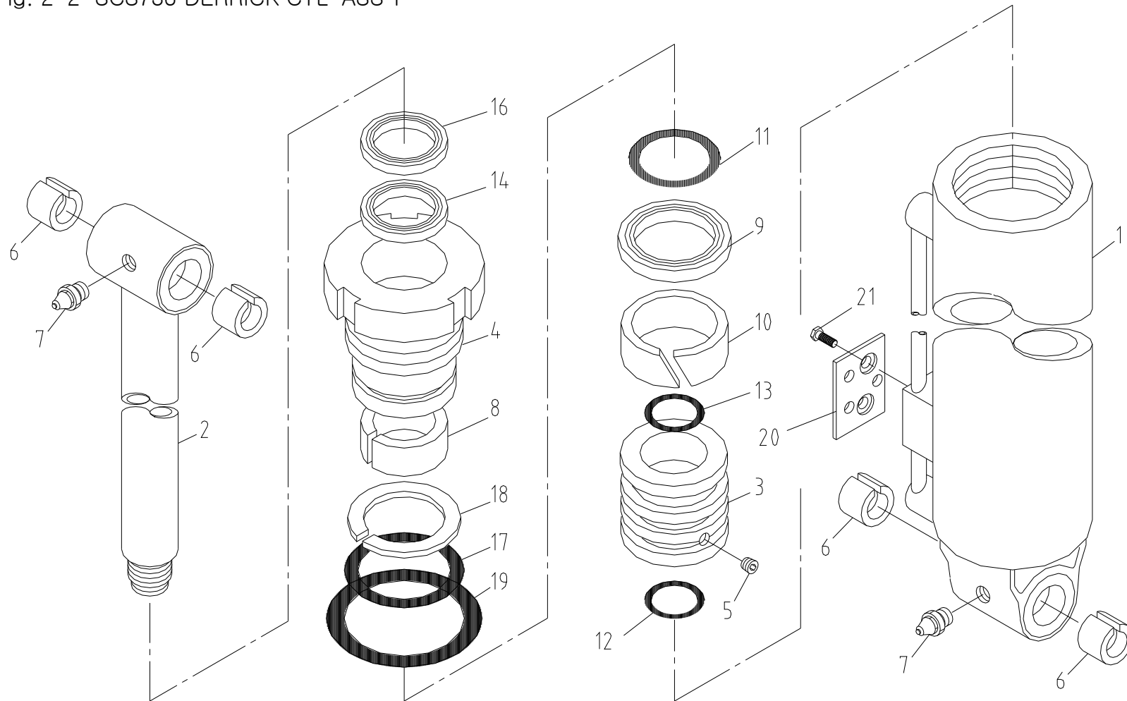
데릭 실린더 조립체 Fig. 2-2 SCS736 DERRICK CYL' ASS'Y
