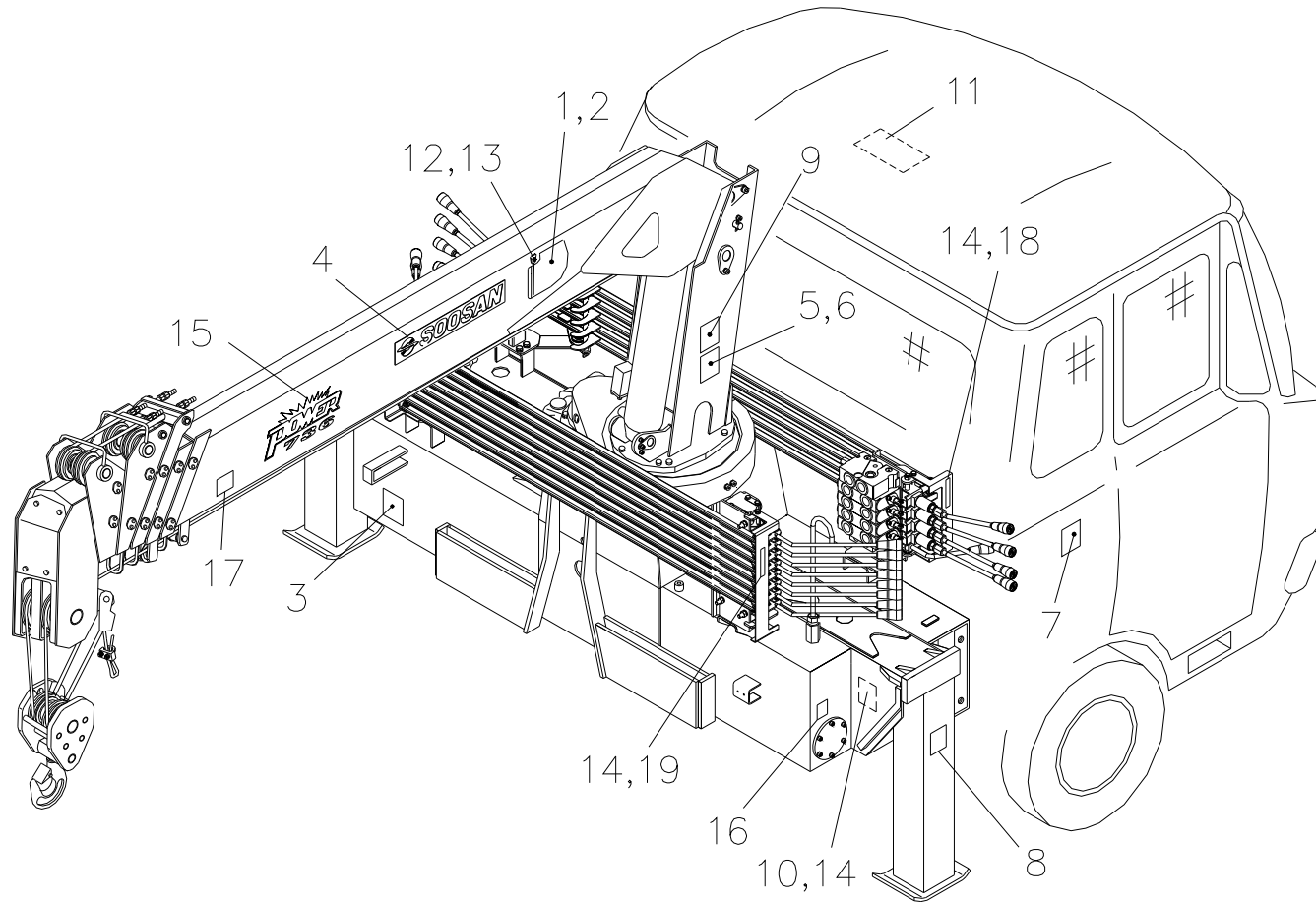
스티커 세트 (표준형)-EXPORT Fig.7 SCS736 STICKER SET (STD)
