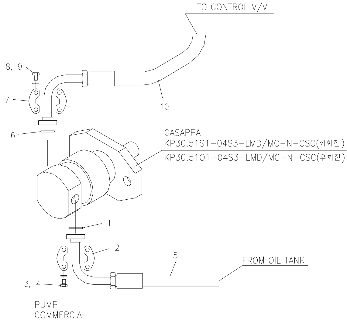
장착 배관 파트 Fig. 8-6 SCS736 M/T PIPING PART
