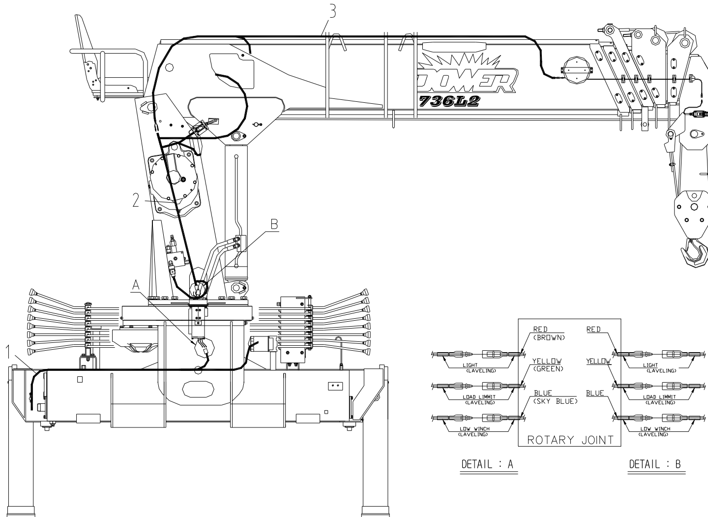
전선 조립체 Fig. 10 SCS736L2 WIRING ASS'Y (TOP)
