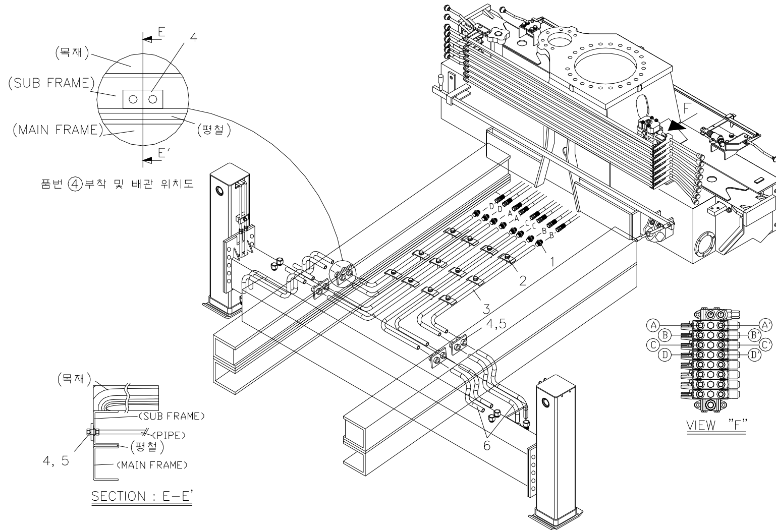
후방 자동 장치 배관 파트 Fig. 8-4 SCS736 R/A M/T PIPING PART
