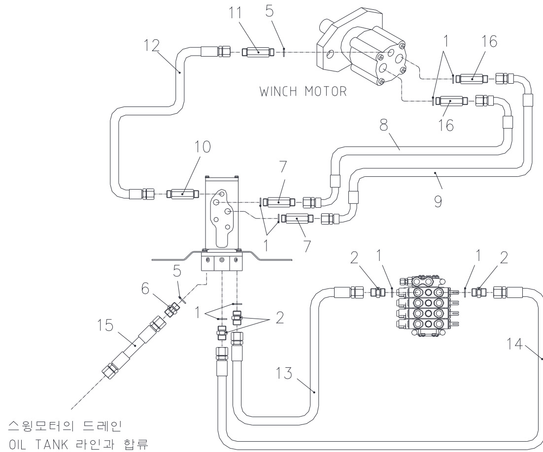
원치 배관 Fig. 5-3 SCS736 WINCH PIPING
