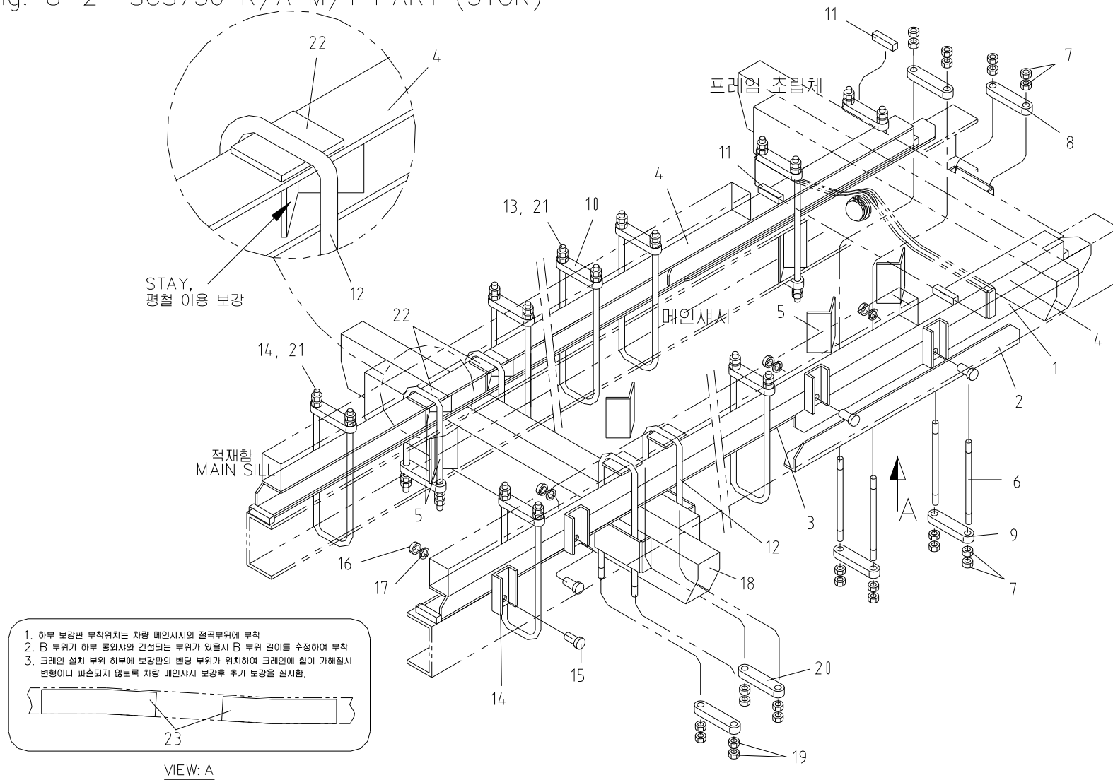
후방 자동 장착 파트 | 5톤 | Fig. 8-2 SCS736 R/A M/T PART (5TON)
