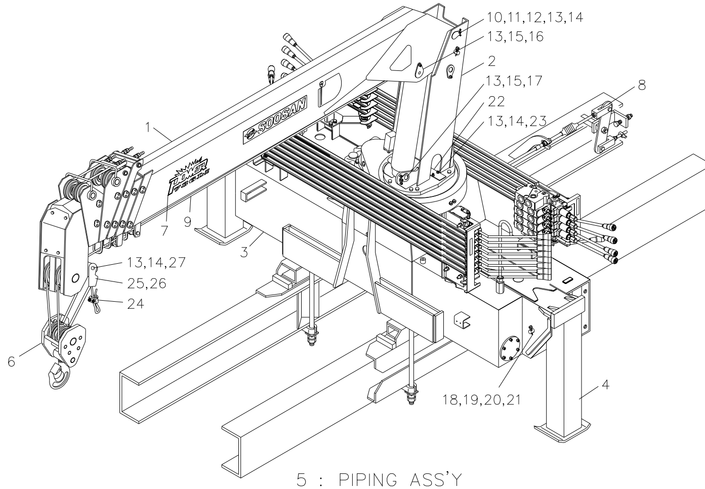
크레인 조립체 (표준형) Fig. 0 SCS736L2 CRANE ASS'Y (STD)
