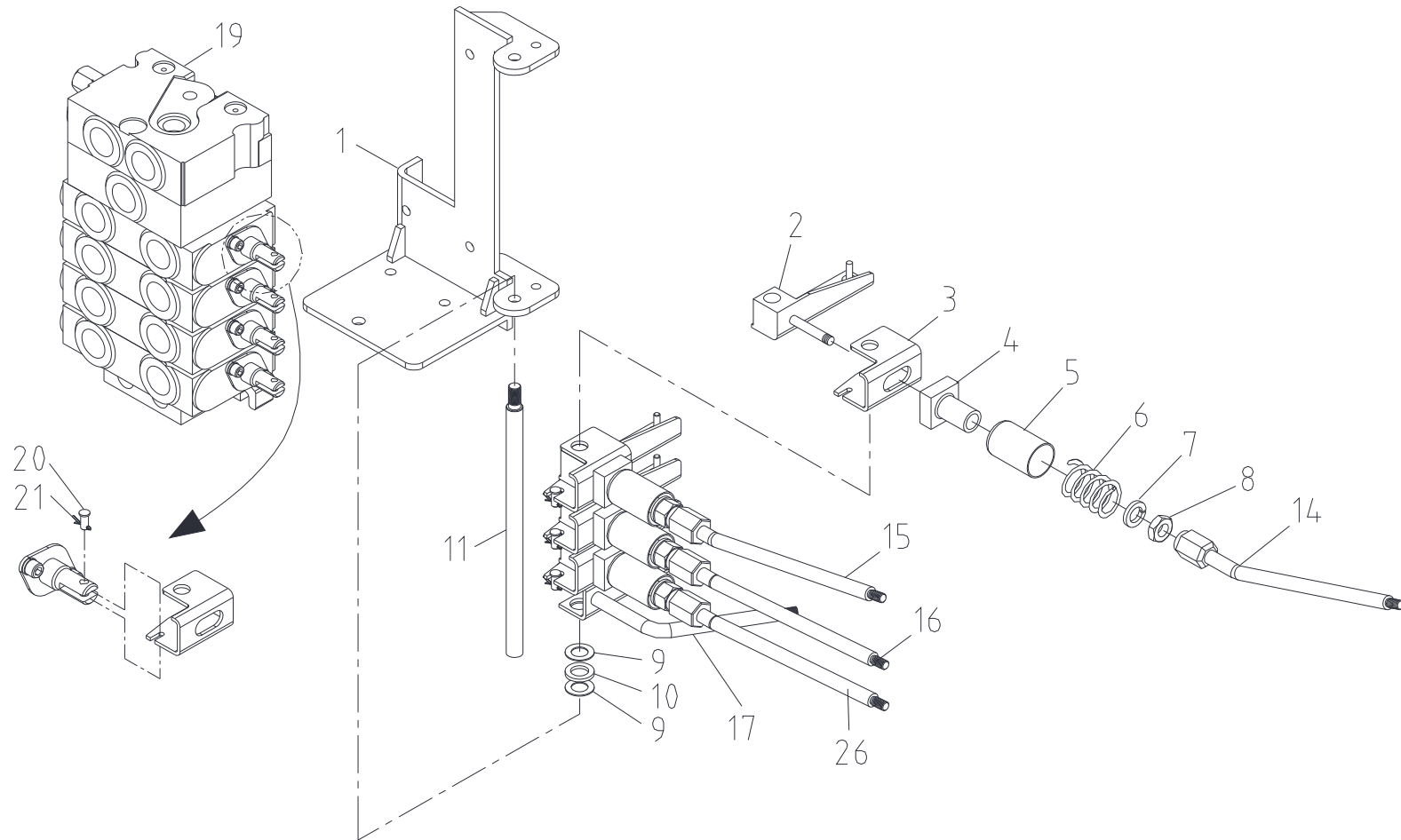
밸브 스탠드 셋 Fig. 3-3-1 SCS736 VALVE STAND SET
