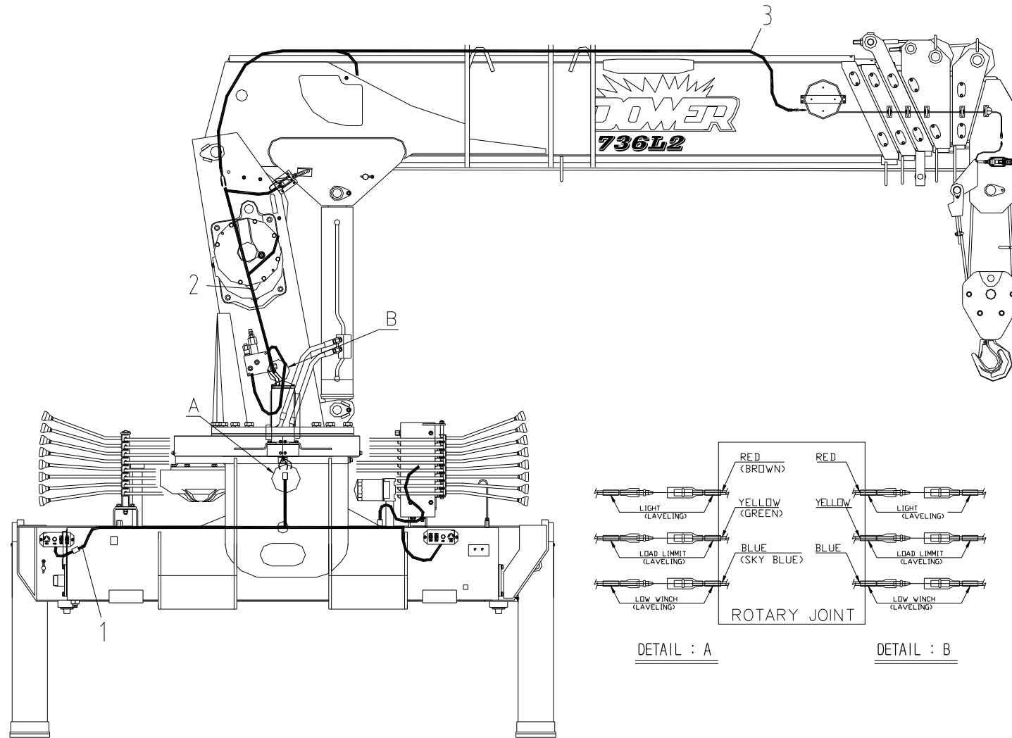
전선 조립체 Fig. 10 SCS736L2 WIRING ASS'Y (STD)
