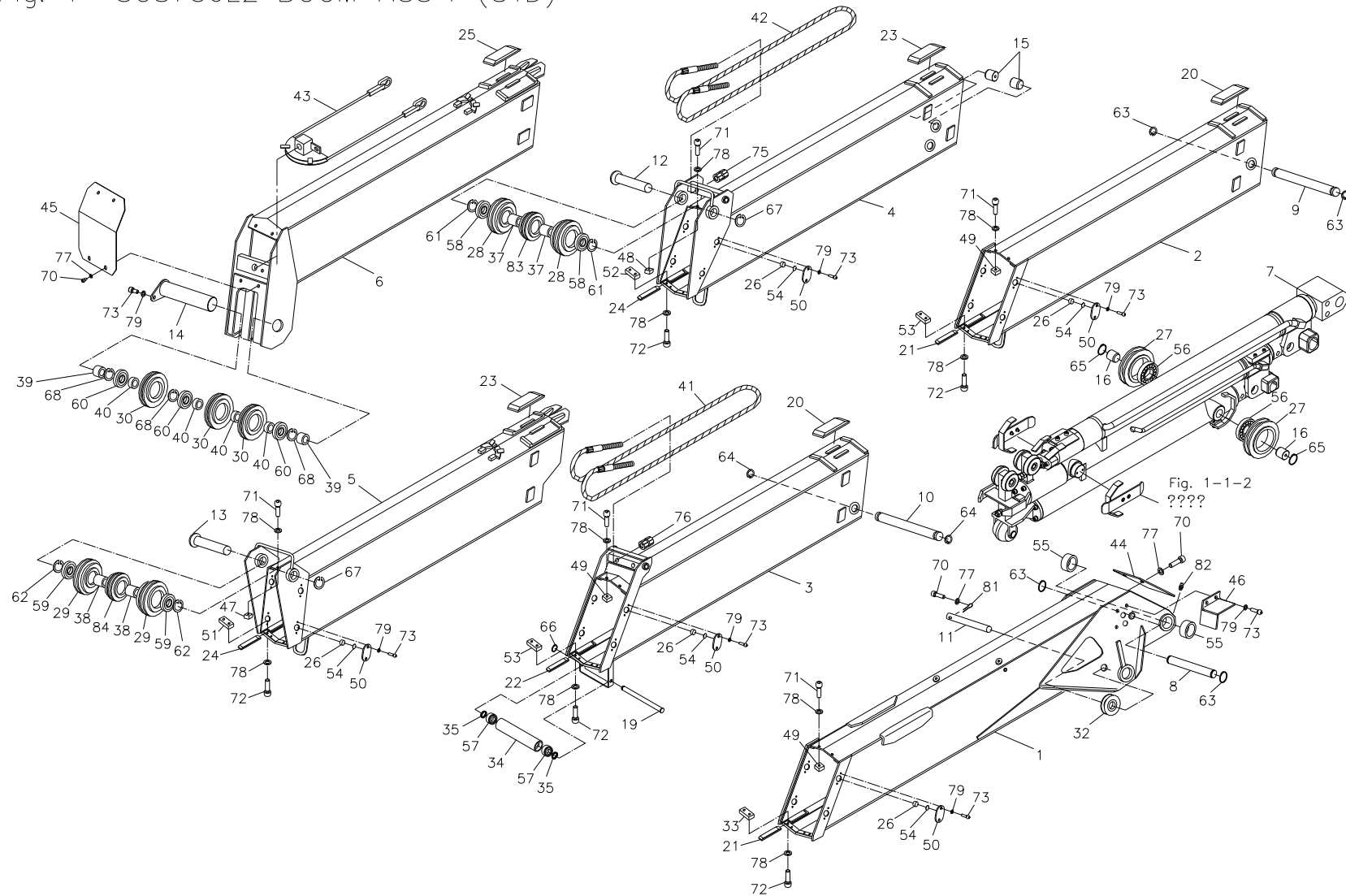
붐 조립체 [표준형] Fig. 1 SCS736L2 BOOM ASS'Y (STD)
