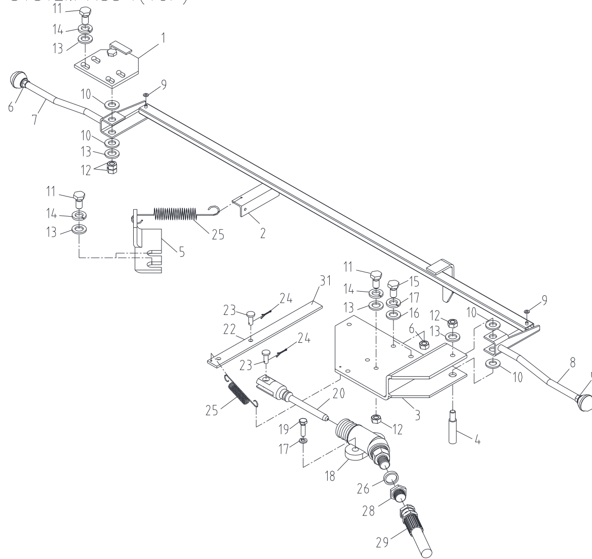
악셀 시스템 조립체(탑형) Fig. 3-3 SCS736 ACC' SYSTEM ASS'Y(TOP)
