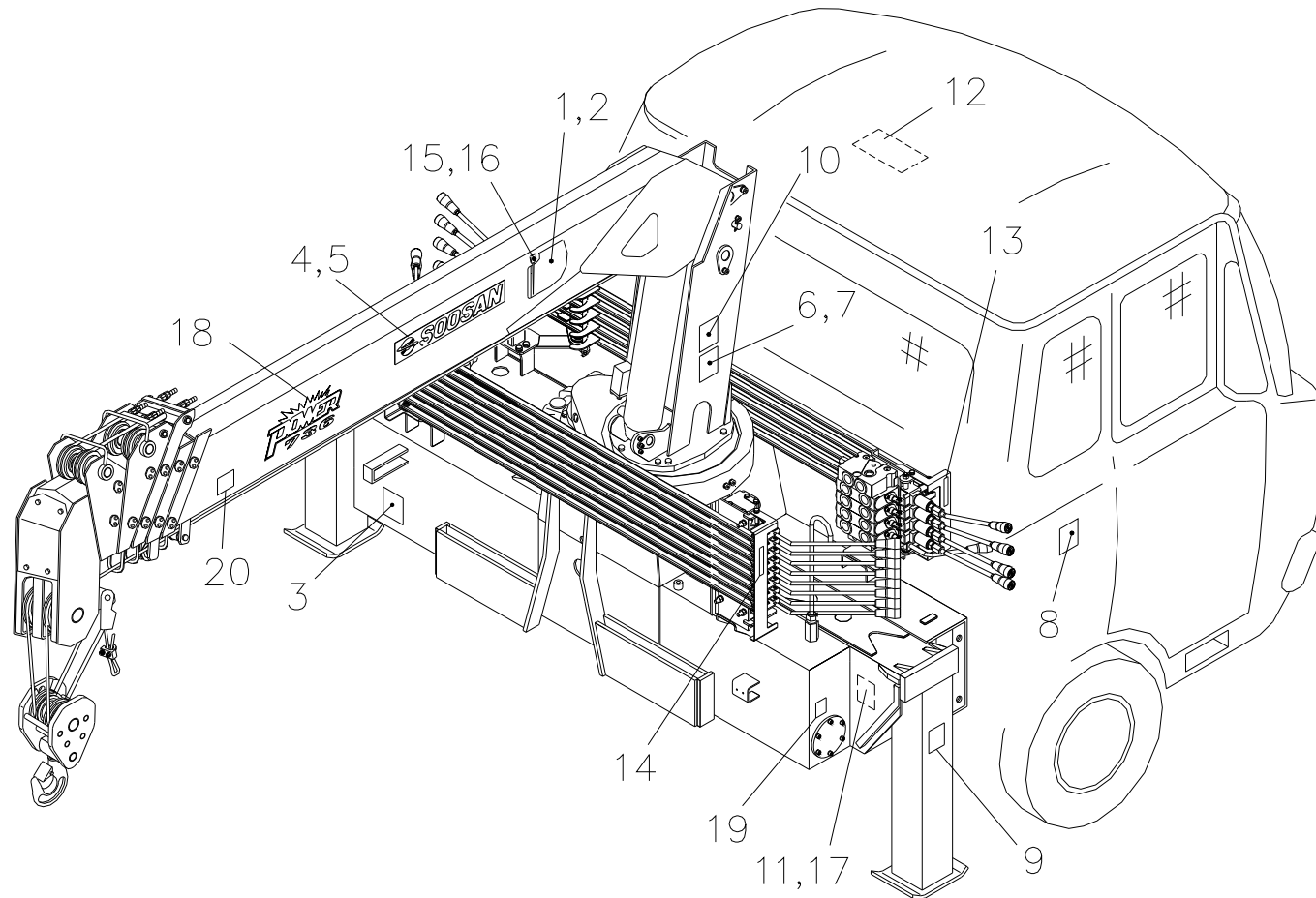
스티커 세트 (표준형)-국내용 Fig.7 SCS736 STICKER SET (STD)
